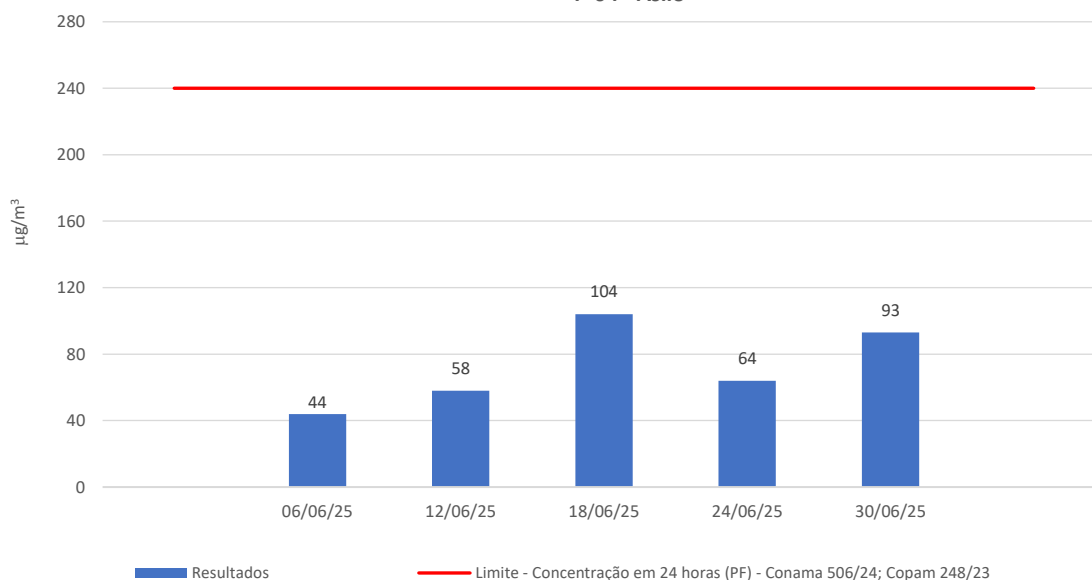
Gráfico 03 - Concentrações de Partículas Totais em Suspensão - PTS P-04 - Asilo
