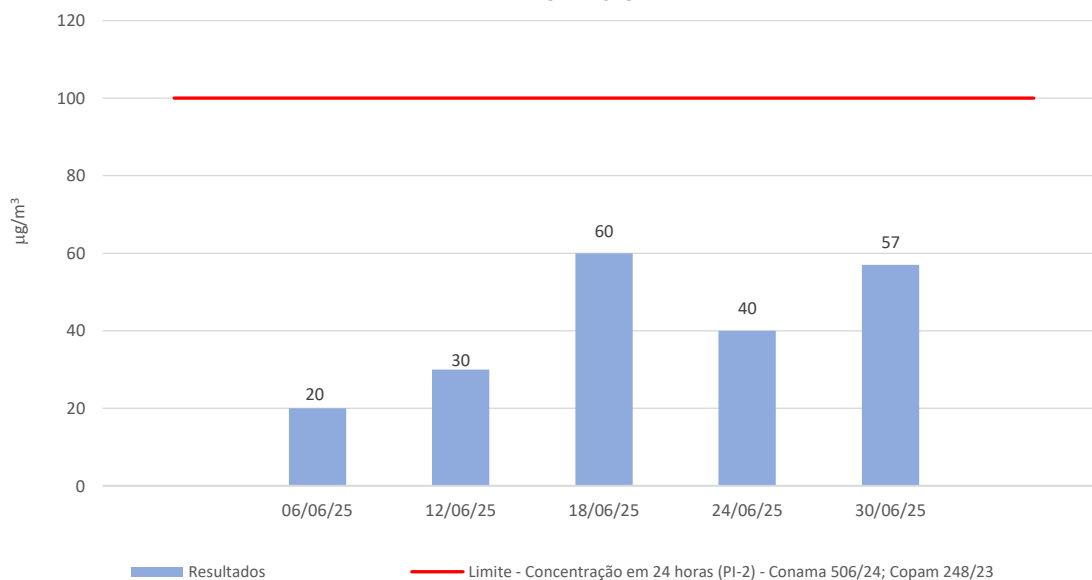
Gráfico 06 - Concentrações de Partículas Inaláveis - PM10 P-04 - Asilo
