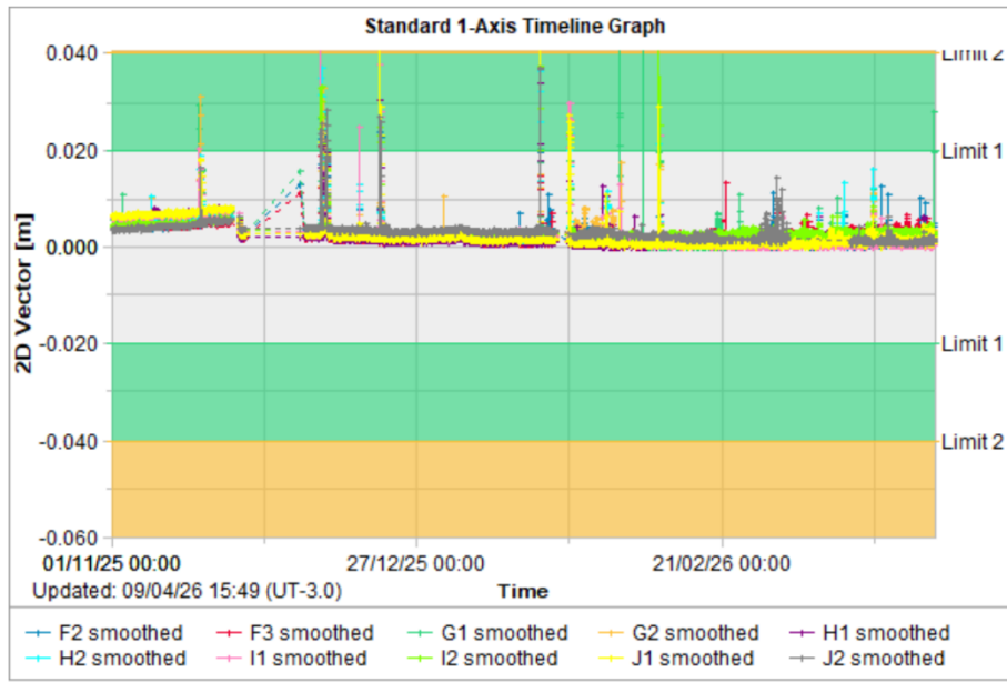
Figura 5.30 – Registros parciais das leituras dos prismas – 2D Vector. (ref: 01/11/25 a 31/03/26)
