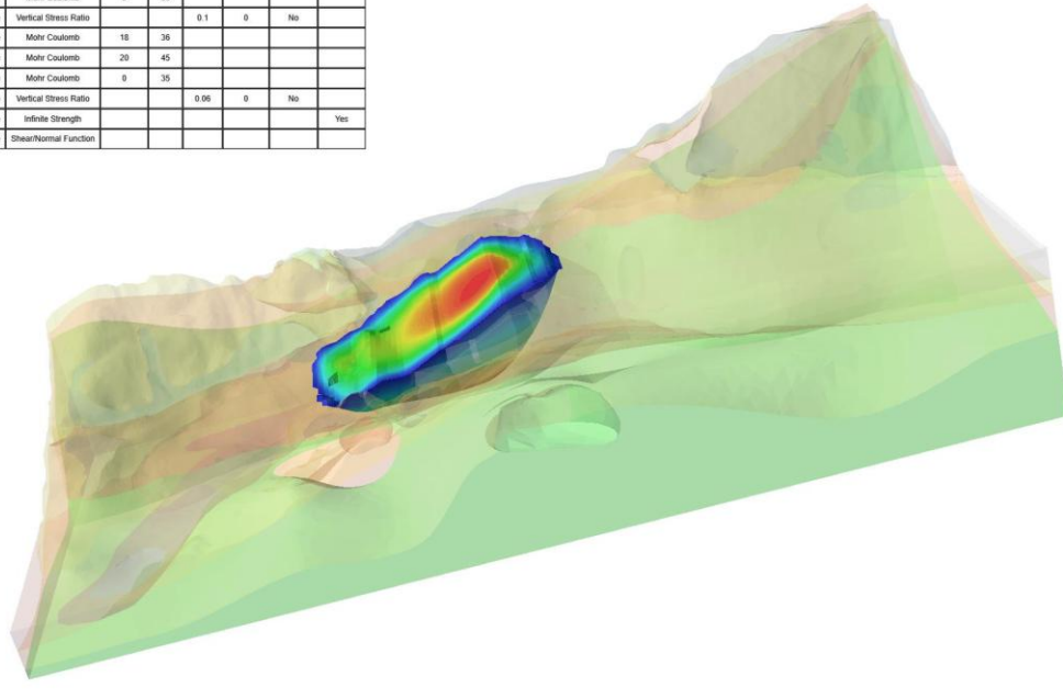
Figura 5.73 – Análise de estabilidade 3D – Rejeitos saturados na condição liquefeita - Vista do mapa de profundidade da superfície de ruptura crítica.
