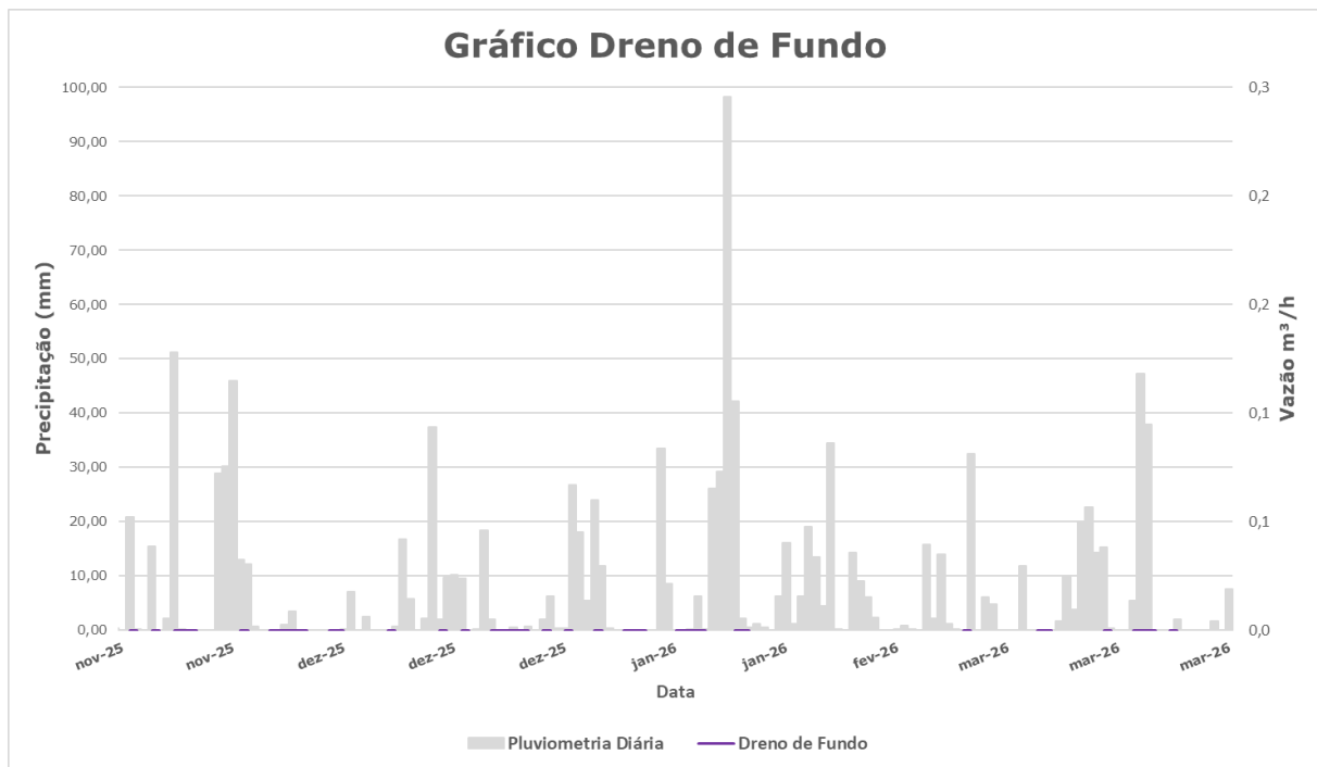
Figura 5.22 – Análise das vazões do IV-01 (Dreno de Fundo).
