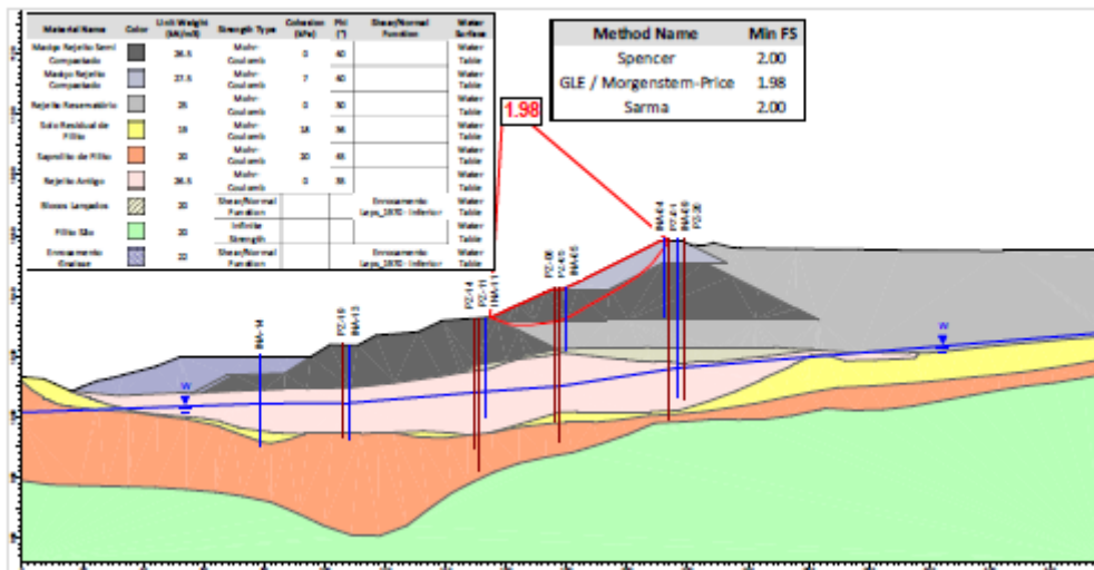
Figura 5.59 – Seção B-B' – Análise Drenada – Superfície de ruptura plano-circular otimizada – Freática 25/02/2026.
