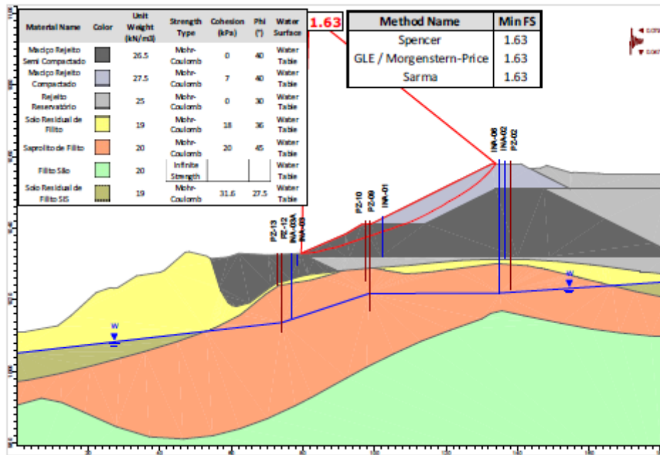
Figura 5.58 – Seção A-A' – Análise Não Drenada – Superfície de ruptura plano-circular otimizada – Freática 25/02/2026 – Razão de resistência não drenada de pico + sismo ↓
