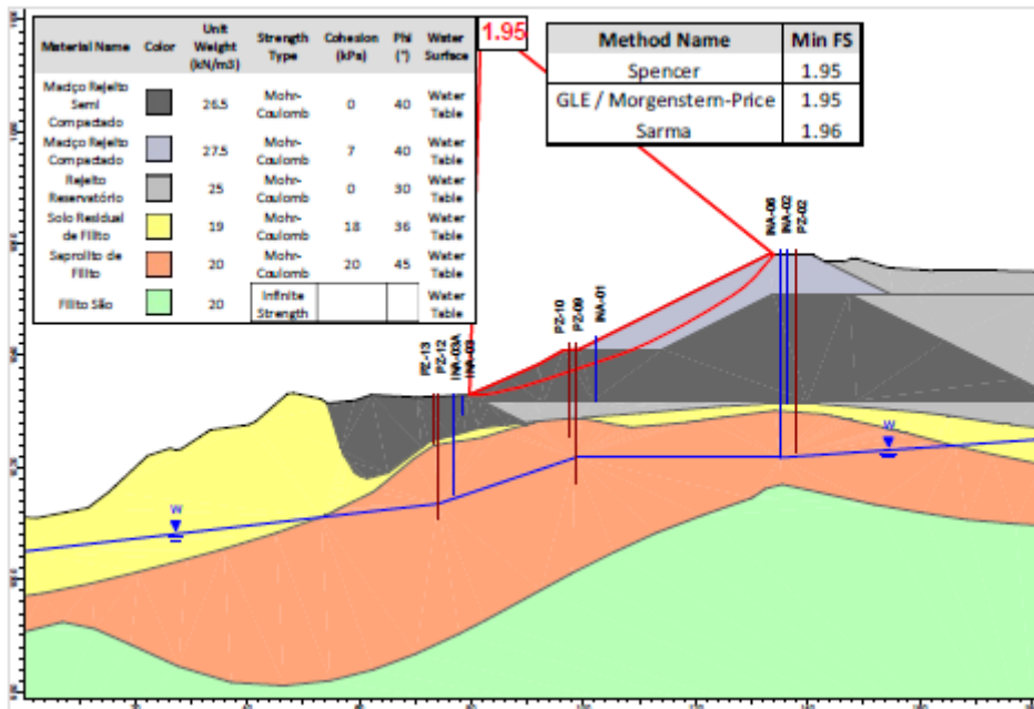
Figura 5.55 – Seção A-A' – Análise Não Drenada – Superfície de ruptura plano-circular otimizada – Freática 25/02/2026 – Razão de resistência não drenada de pico.
