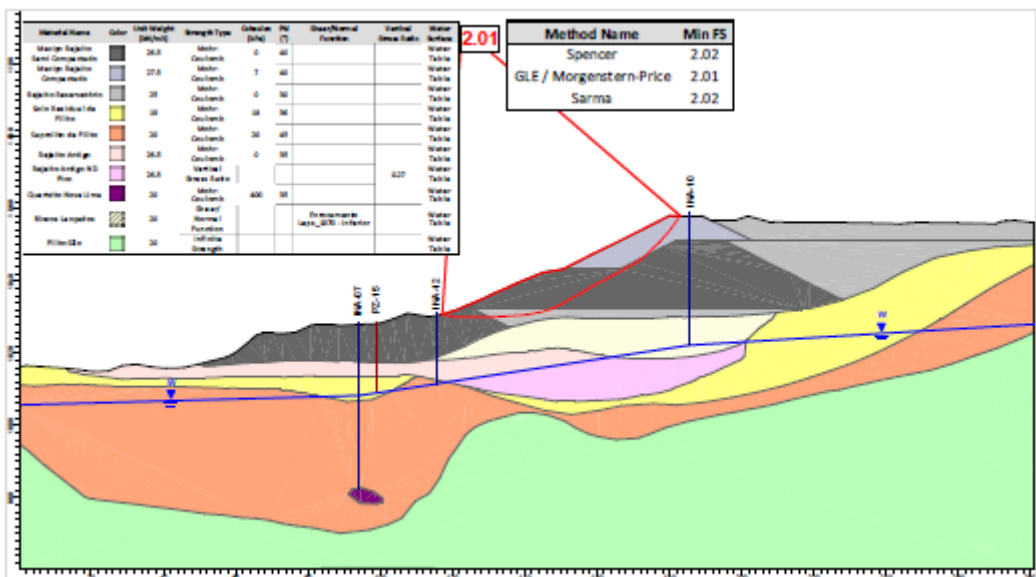
Figura 5.65 – Seção C-C' – Análise Não Drenada – Superfície de ruptura plano-circular otimizada – Freática 25/02/2026 – Razão de resistência não drenada de pico.
