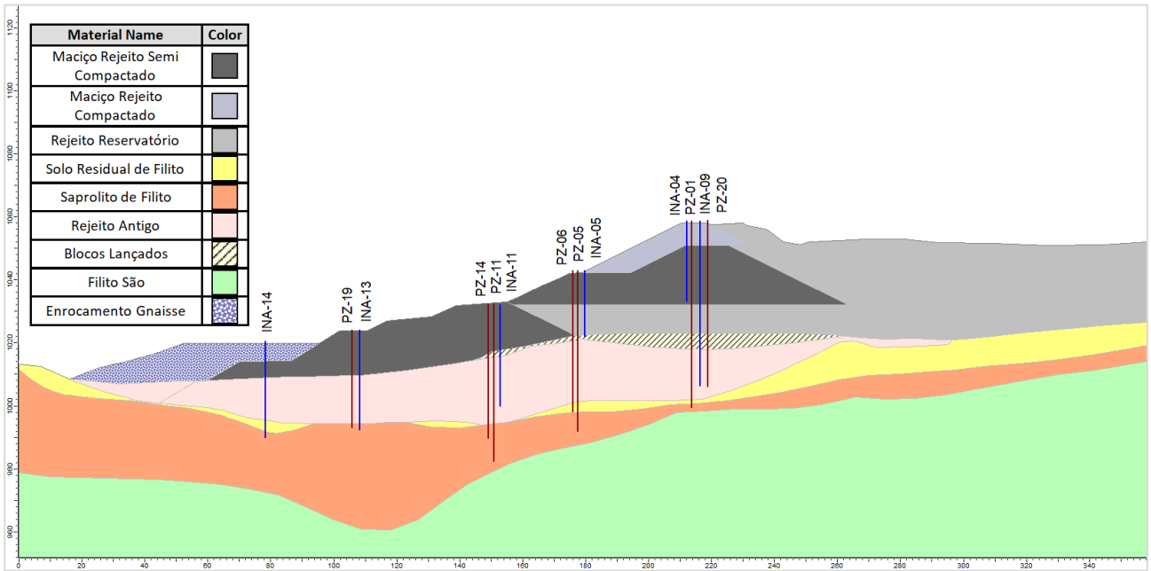
Figura 5.16 – Seção transversal de controle B-B'.
