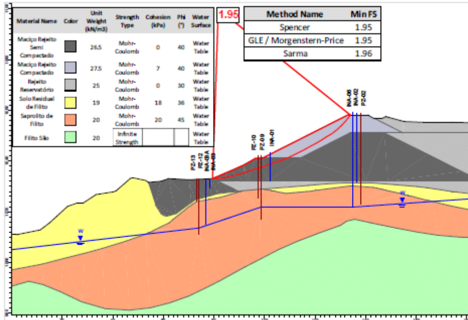
Figura 5.56 – Seção A-A' – Análise Não Drenada – Superfície de ruptura plano-circular otimizada – Freática 25/02/2026 – Razão de resistência não drenada liquefeita.
