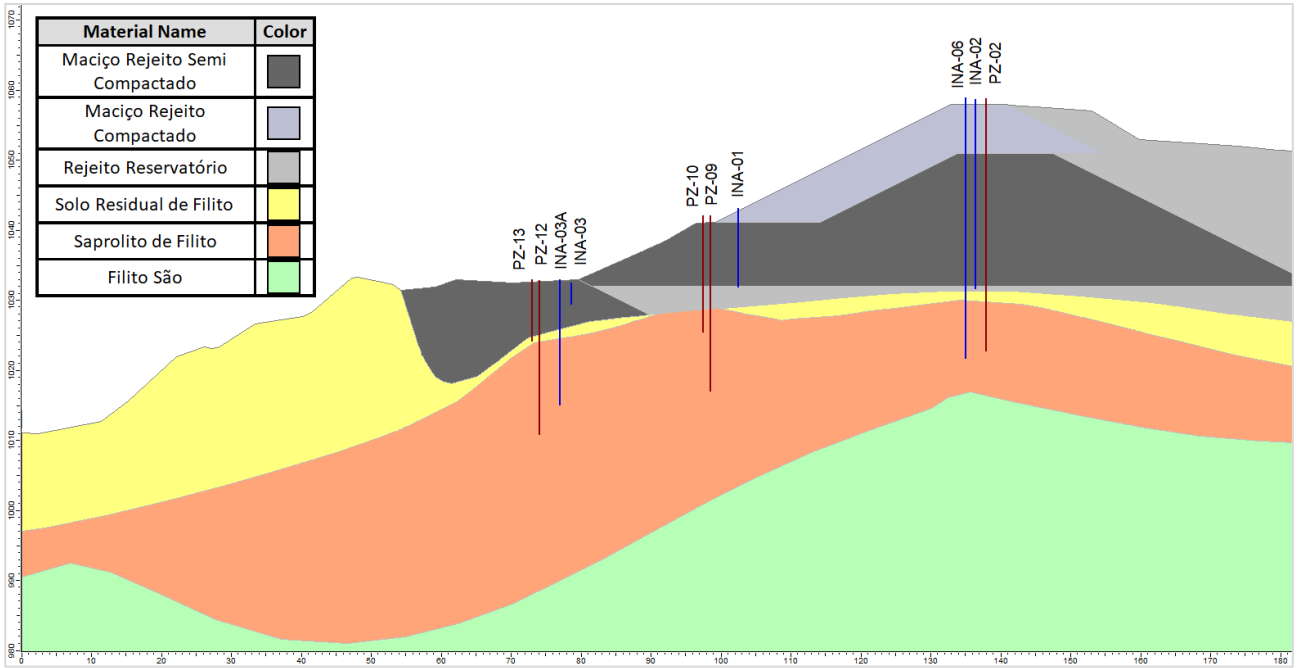
Figura 5.15 – Seção transversal de controle A-A'.
