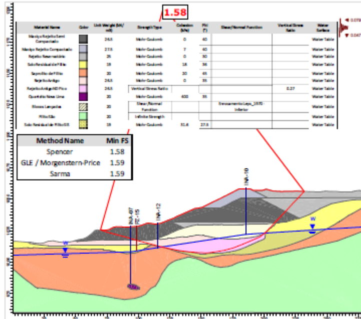
Figura 5.68 – Seção C-C’ – Análise Não Drenada – Superfície de ruptura plano-circular otimizada – Freática 25/02/2026 – Razão de resistência não drenada de pico + sismo ↓
