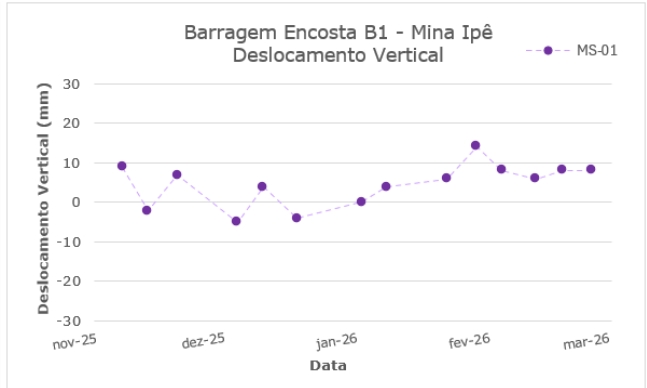
Figura 5.35 – Prisma de monitoramento da encosta MS-01.
