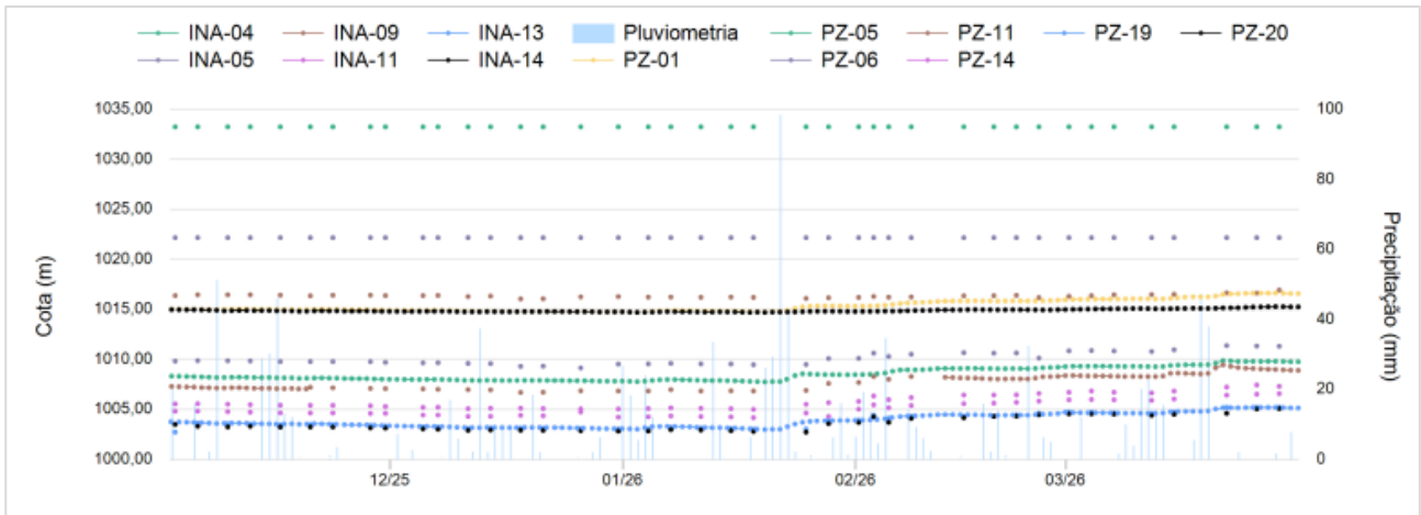
Figura 5.19 - Instrumentos Seção B-B
