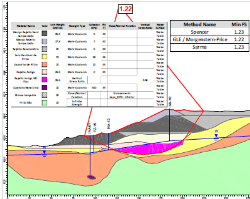
Figura 5.66 – Seção C-C' – Análise Não Drenada – Superfície de ruptura plano-circular otimizada – Freática 25/02/2026 – Razão de resistência não drenada liquefeito.
