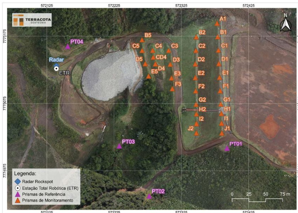
Figura 5.24 - Localização dos prismas instalados no maciço da Barragem B1 – Mina Ipê.
