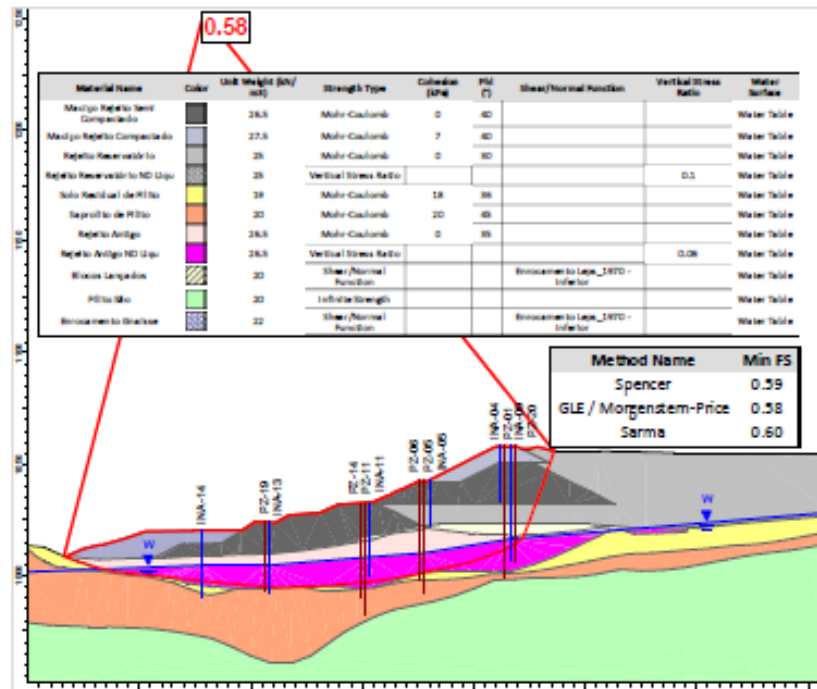
Figura 5.61 – Seção B-B' – Análise Não Drenada – Superfície de ruptura plano-circular otimizada – Freática 25/02/2026 – Razão de resistência não drenada liquefeito.
