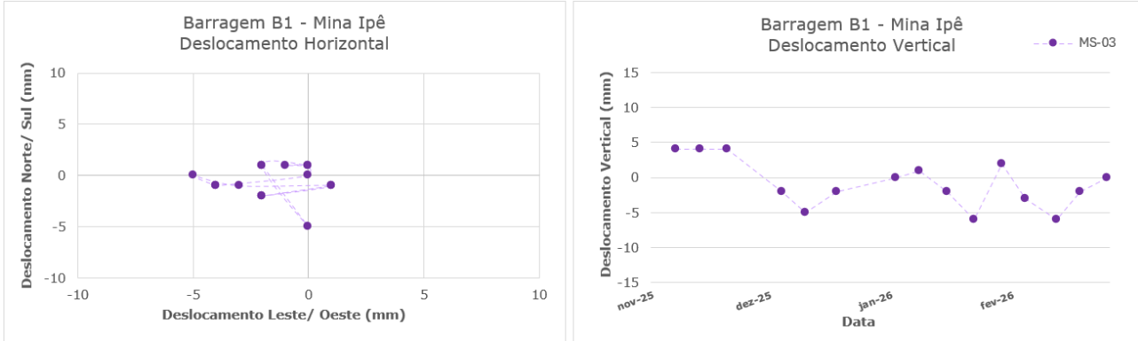
Figura 5.33 – Marco de controle de deformação – MS-03.
