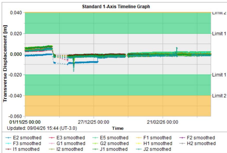
Figura 5.28 – Registros parciais das leituras dos prismas – Transverse Displacement. (ref: 01/11/25 a 31/03/26)
