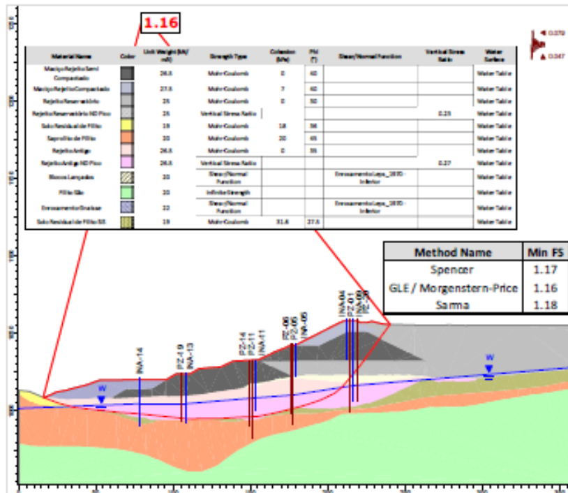
Figura 5.62 – Seção B-B’ – Análise Não Drenada – Superfície de ruptura plano-circular otimizada – Freática 25/02/2026– Razão de resistência não drenada de pico + sismo ↑.
