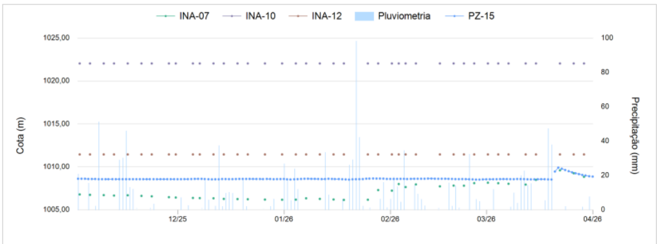
Figura 5.20 - Instrumentos Seção C-C.
