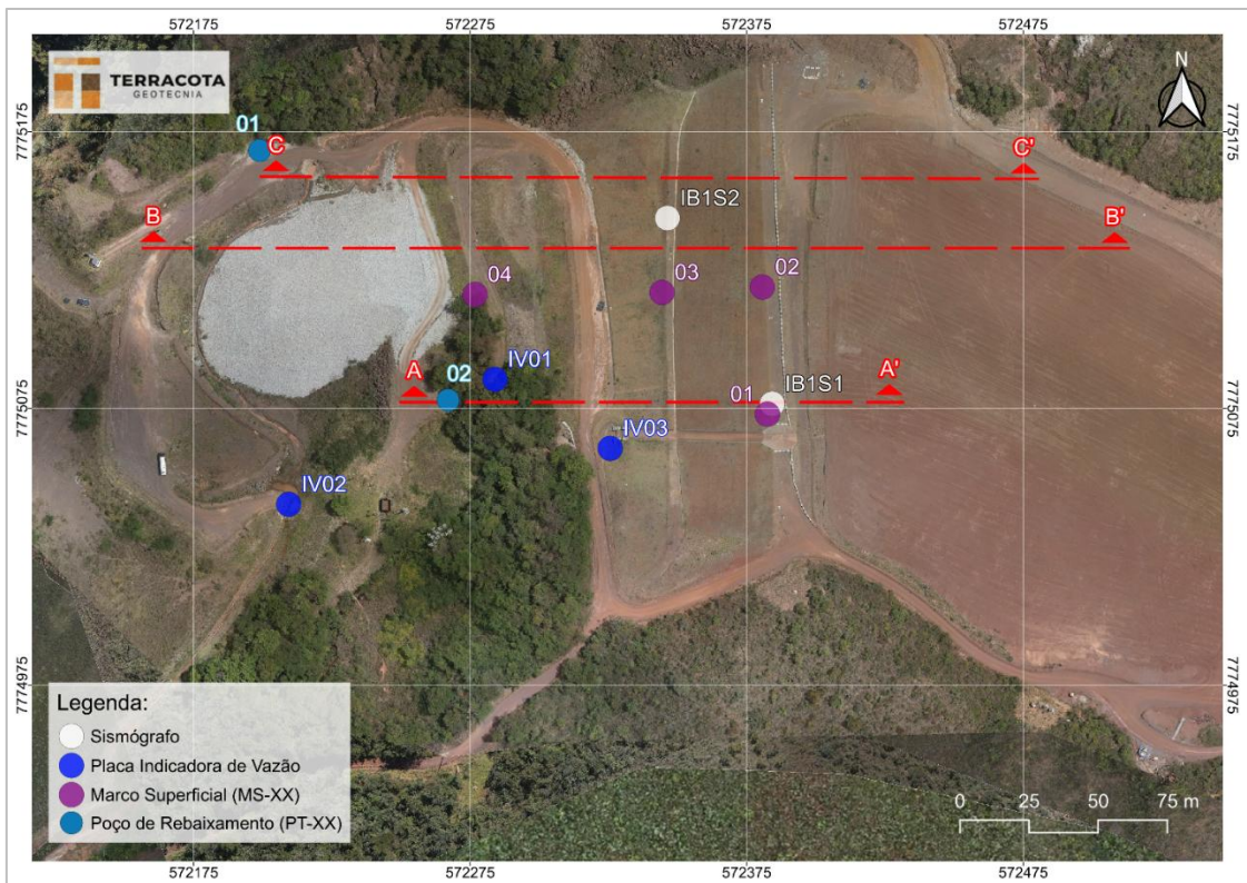
Figura 5.14 – Localização Marcos Superficiais, Sismógrafos e Placas Indicadoras de Vazão – Barragem B1 – Mina Ipê.
