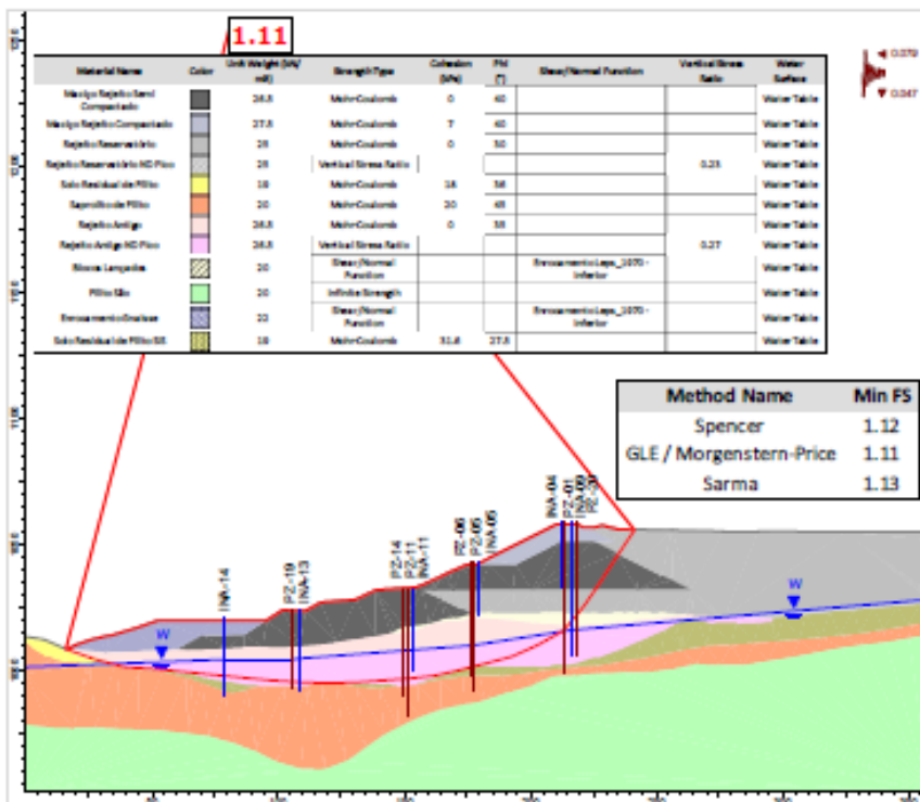
Figura 5.63 – Seção B-B’ – Análise Não Drenada – Superfície de ruptura plano-circular otimizada – Freática 25/02/2026 – Razão de resistência não drenada de pico + sismo ↓.
