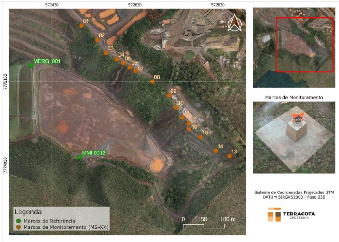
Figura 5.11 - Localização dos marcos instalados para monitoramento da encosta na margem direita do reservatório da Barragem B1 – Mina Ipê.
