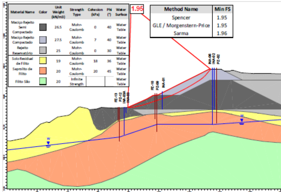
Figura 5.54 – Seção A-A' – Análise Drenada – Superfície de ruptura plano-circular otimizada – Freática 25/02/2026.
