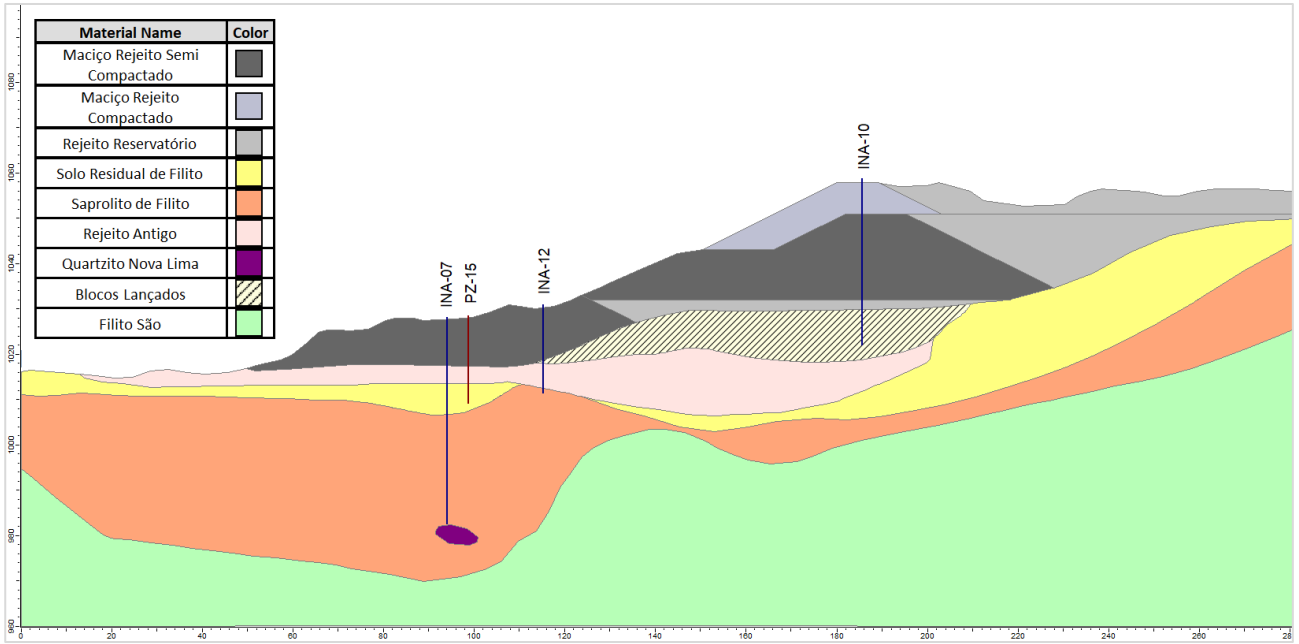
Figura 5.17 – Seção transversal de controle C-C’.
