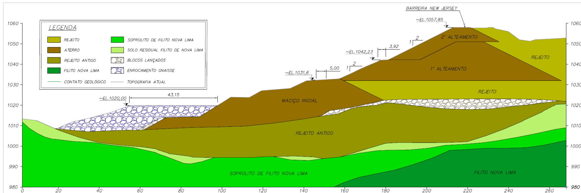
Figura 4.3 – Seção de maior altura B-B' da Barragem B1 – Mina Ipê.
