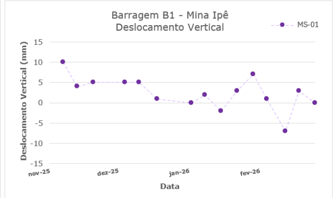
Figura 5.31 – Marco de controle de deformação – MS-01.
