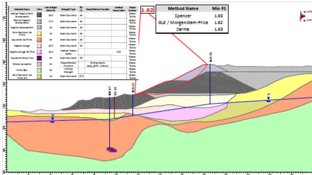
Figura 5.67 – Seção C-C' – Análise Não Drenada – Superfície de ruptura plano-circular otimizada – Freática 25/02/2026 – Razão de resistência não drenada de pico + sismo ↑
