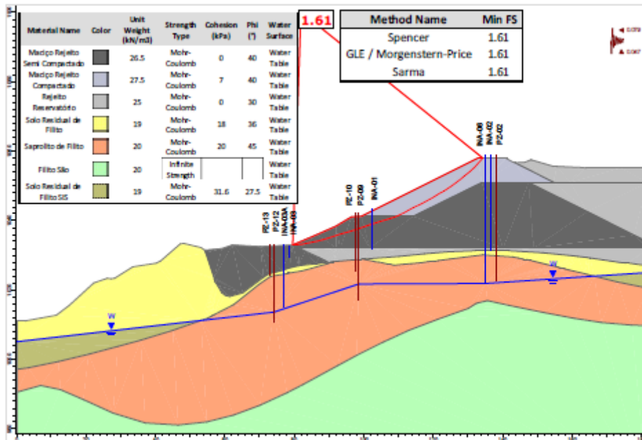
Figura 5.57 – Seção A-A' – Análise Não Drenada – Superfície de ruptura plano-circular otimizada – Freática 25/02/2026 – Razão de resistência não drenada de pico + sismo ↑ .
