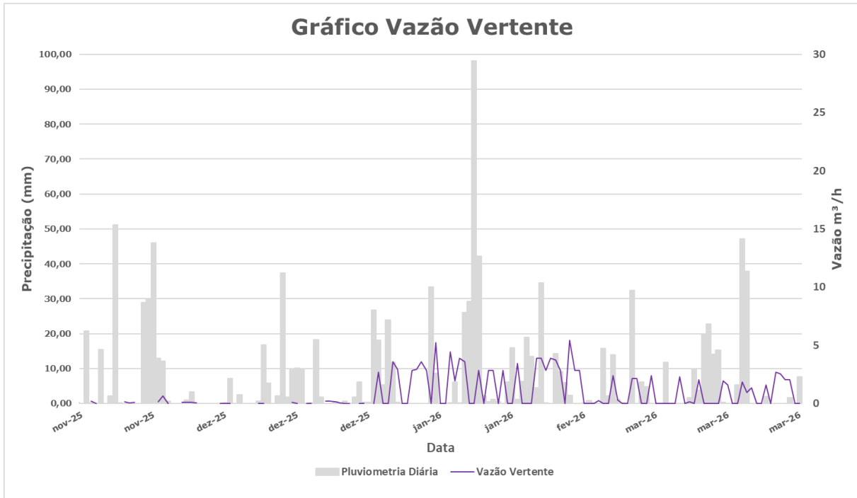
Figura 5.23 – Análise das vazões do IV-02 (Vertente).
