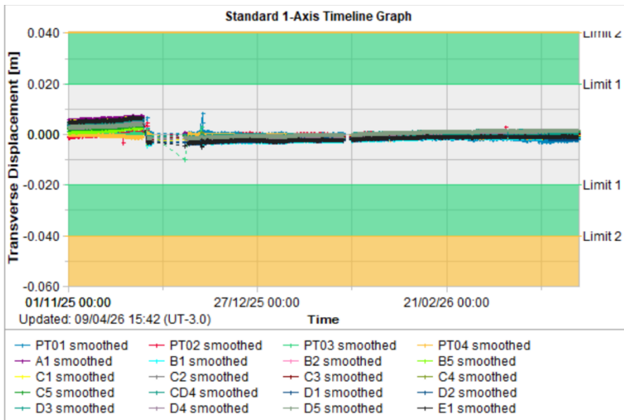
Figura 5.27 – Registros parciais das leituras dos prismas – Transverse Displacement. (ref: 01/11/25 a 31/03/26)
