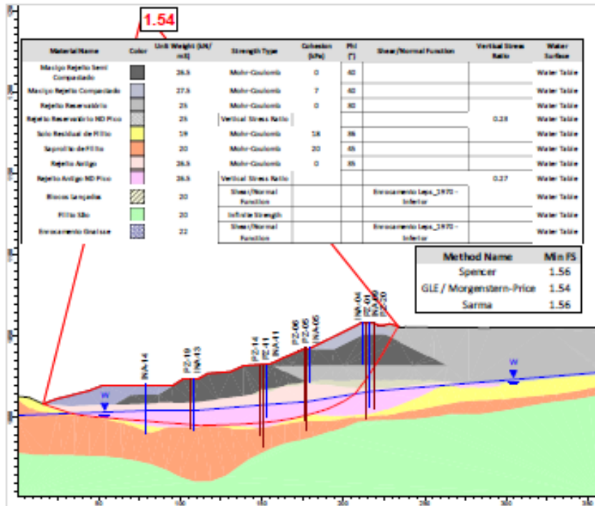
Figura 5.60 – Seção B-B' – Análise Não Drenada – Superfície de ruptura plano-circular otimizada – Freática 25/02/2026 – Razão de resistência não drenada de pico.
