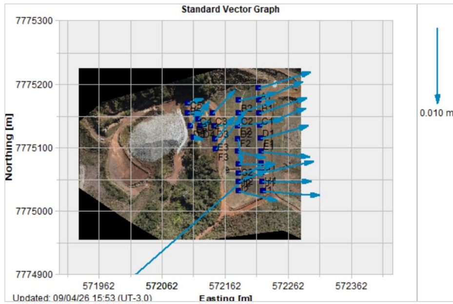
Figura 5.26 – Registros vetores deslocamento dos prismas. (ref: 01/11/25 a 31/03/26)
