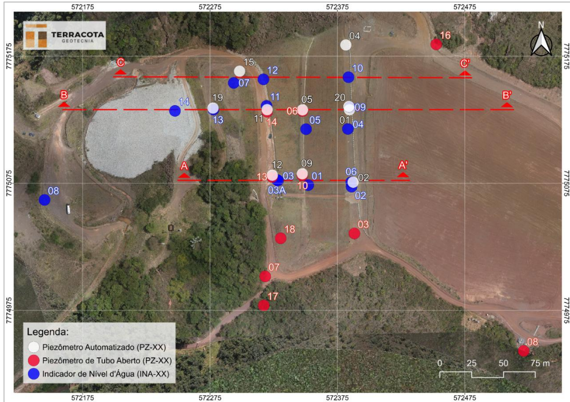
Figura 5.13 – Localização dos INA's e PZ's – Barragem B1 – Mina Ipê.
