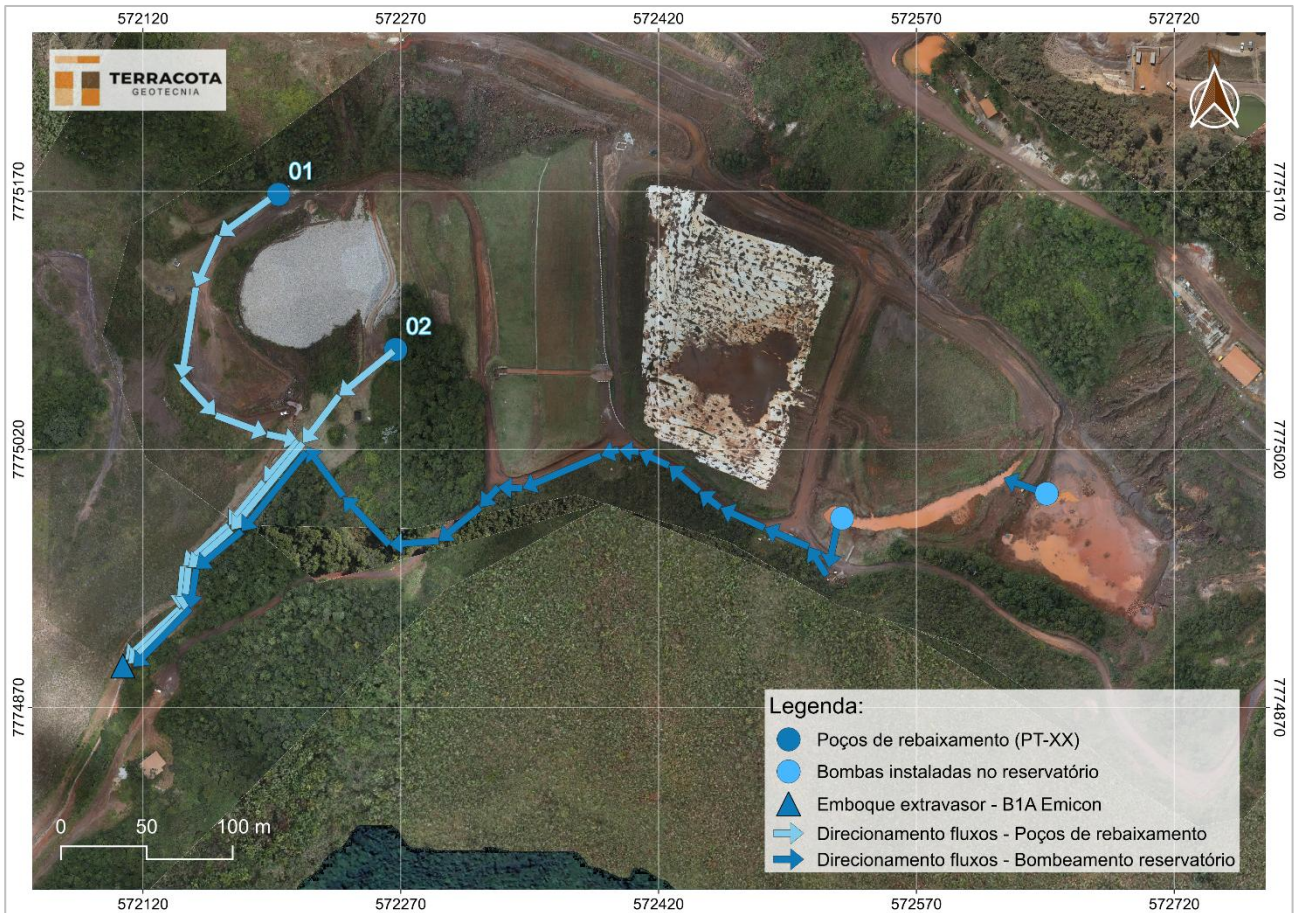
Figura 5.49 – Esquema de direcionamento atual dos fluxos proveniente dos sistemas de bombeamento.
