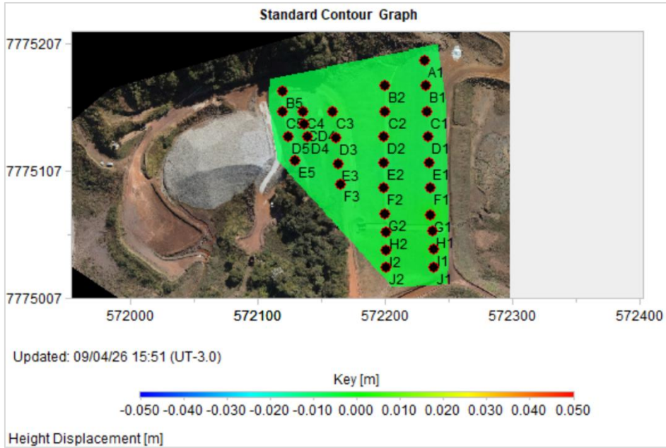
Figura 5.25 – Registros deslocamentos verticais dos prismas. (ref: 01/11/25 a 31/03/26)
