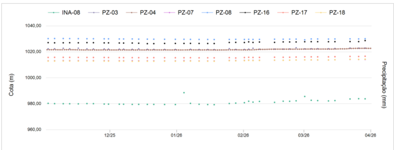
Figura 5.21 - Instrumentos Sem Seção.
