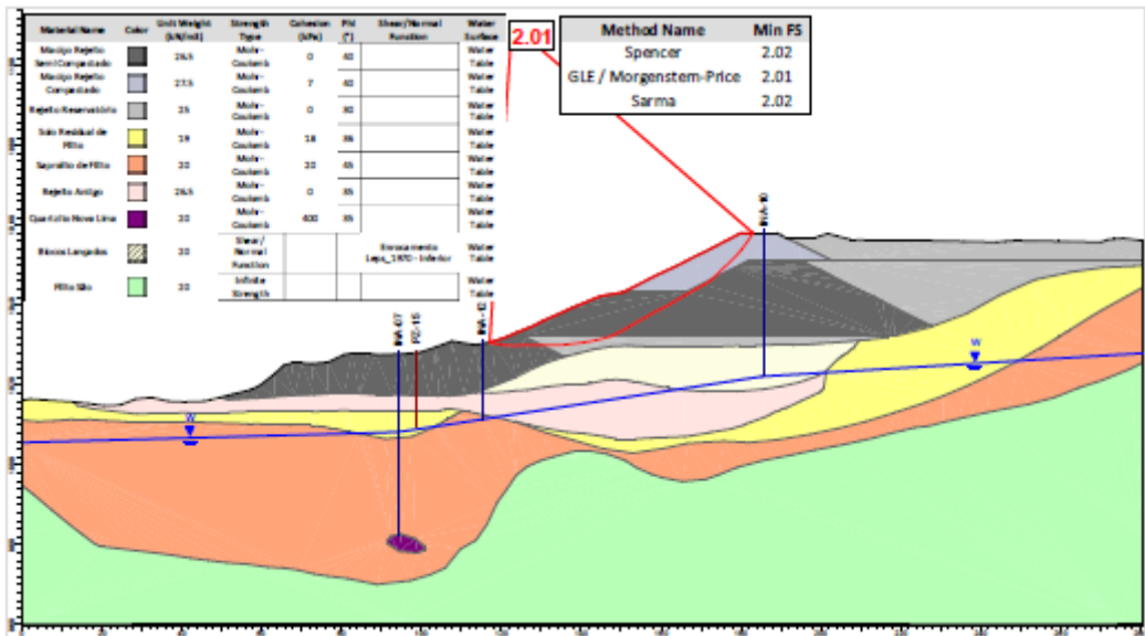
Figura 5.64 – Seção C-C' – Análise Drenada – Superfície de ruptura plano-circular otimizada – Freática 25/02/2026.
